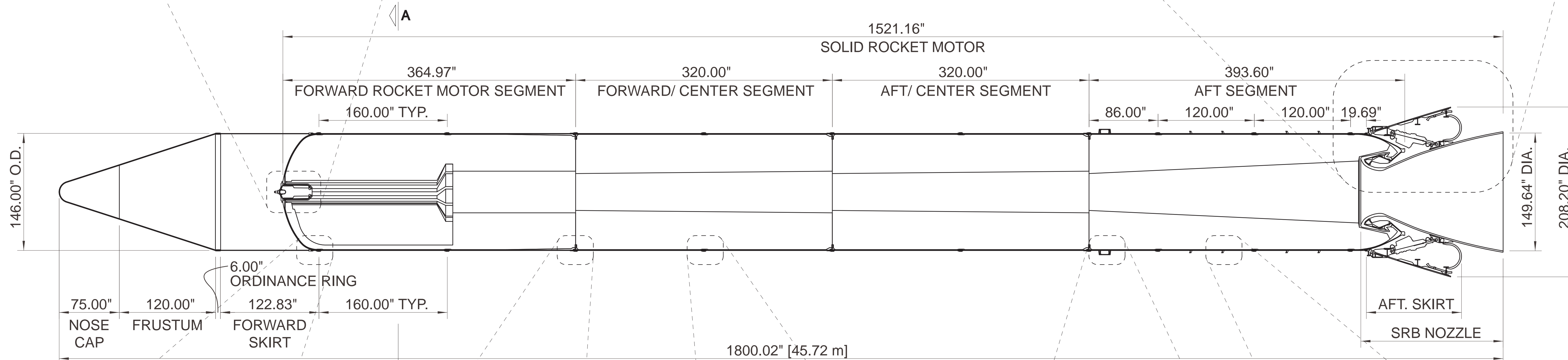
SRB LONGITUDINAL SECTION SCALE: 3/16" = 1'-0"
