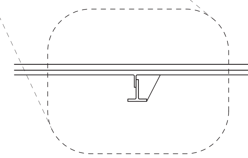
CASE STIFFENER RINGS SCALE: 2" = 1'-0"
